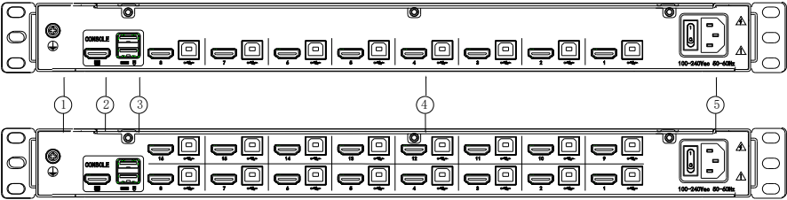
图 2-1.3 后视图
