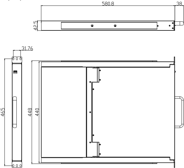
图 1-1.2 17"KVM 尺寸图
